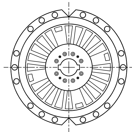
Modalità di fissaggio sull'albero Modality of on-shaft mounting
